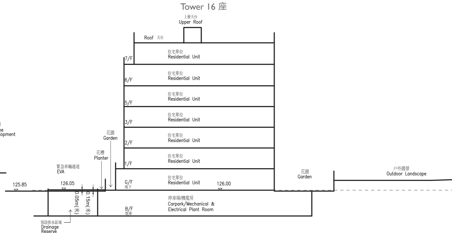
Cross-Section Plan 14 橫截面圖 14
