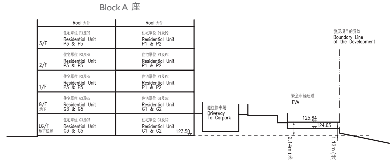
Cross-Section Plan A3 橫截面圖 A3
