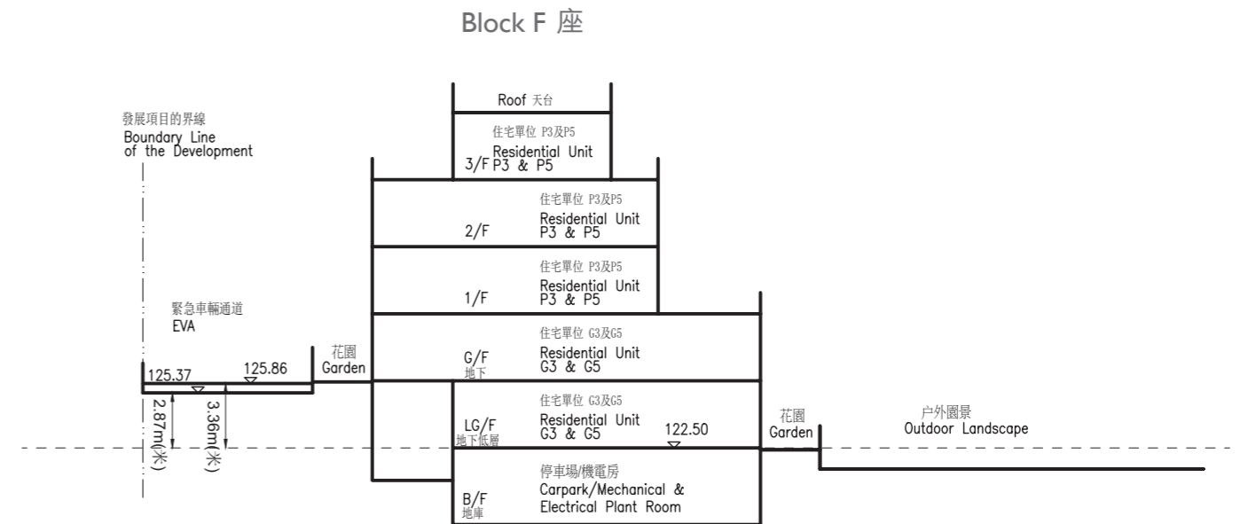
Cross-Section Plan F2 橫截面圖 F2
